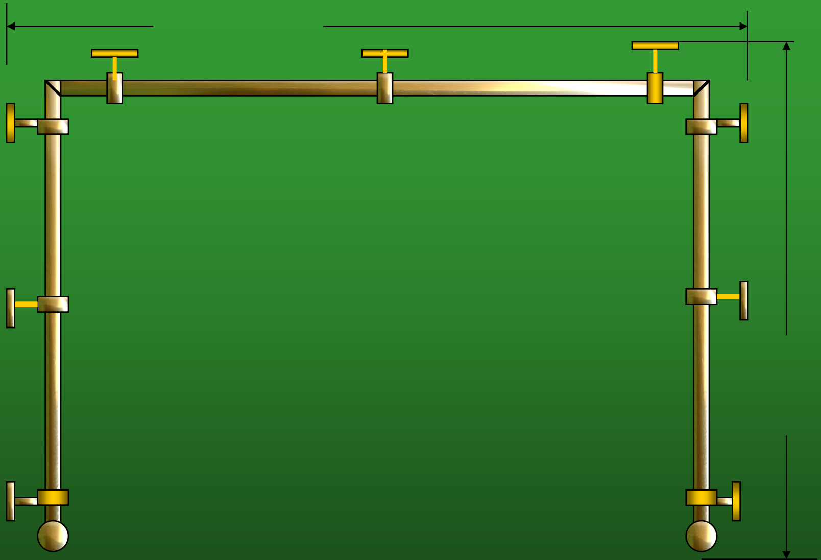
Barra en "U" con Soporte Terminal de Bolo / Piña y unión de 45°
